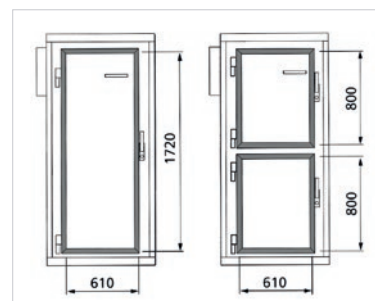
Dimensiones puertas
